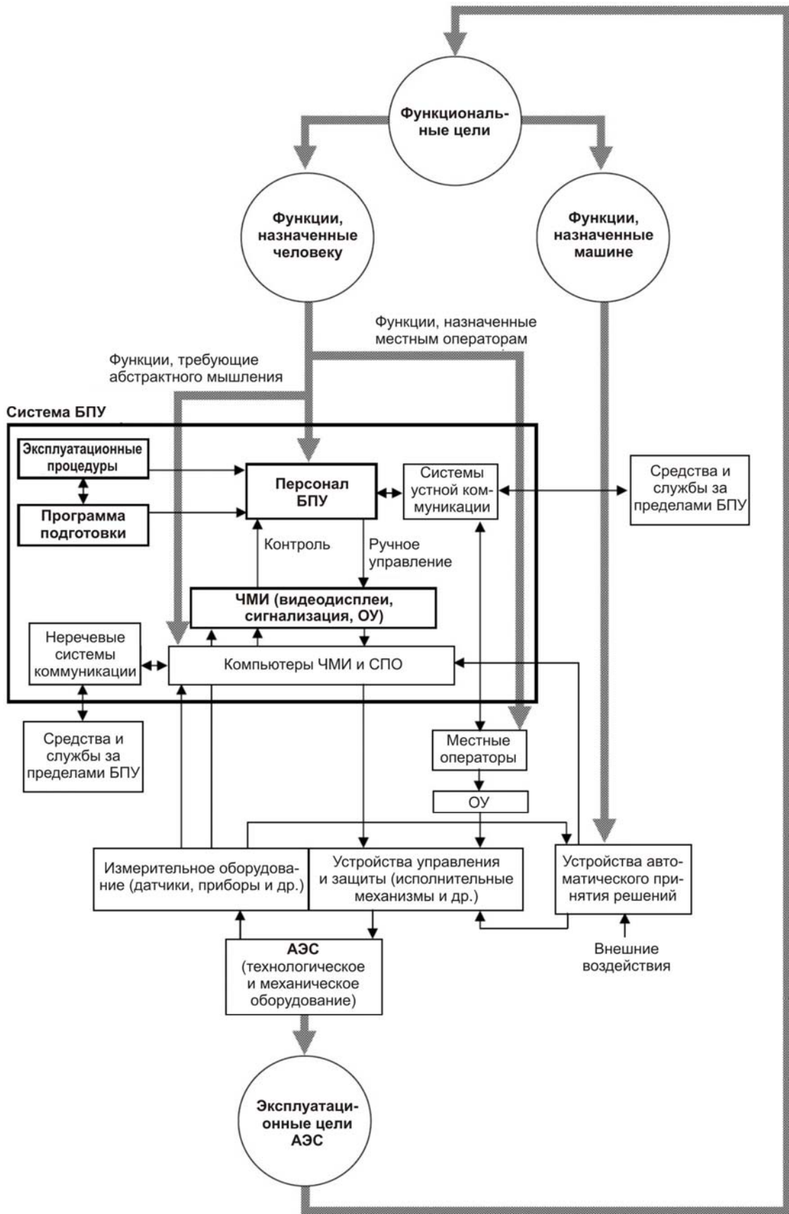
Рисунок 1 — Структура системы БПУ
