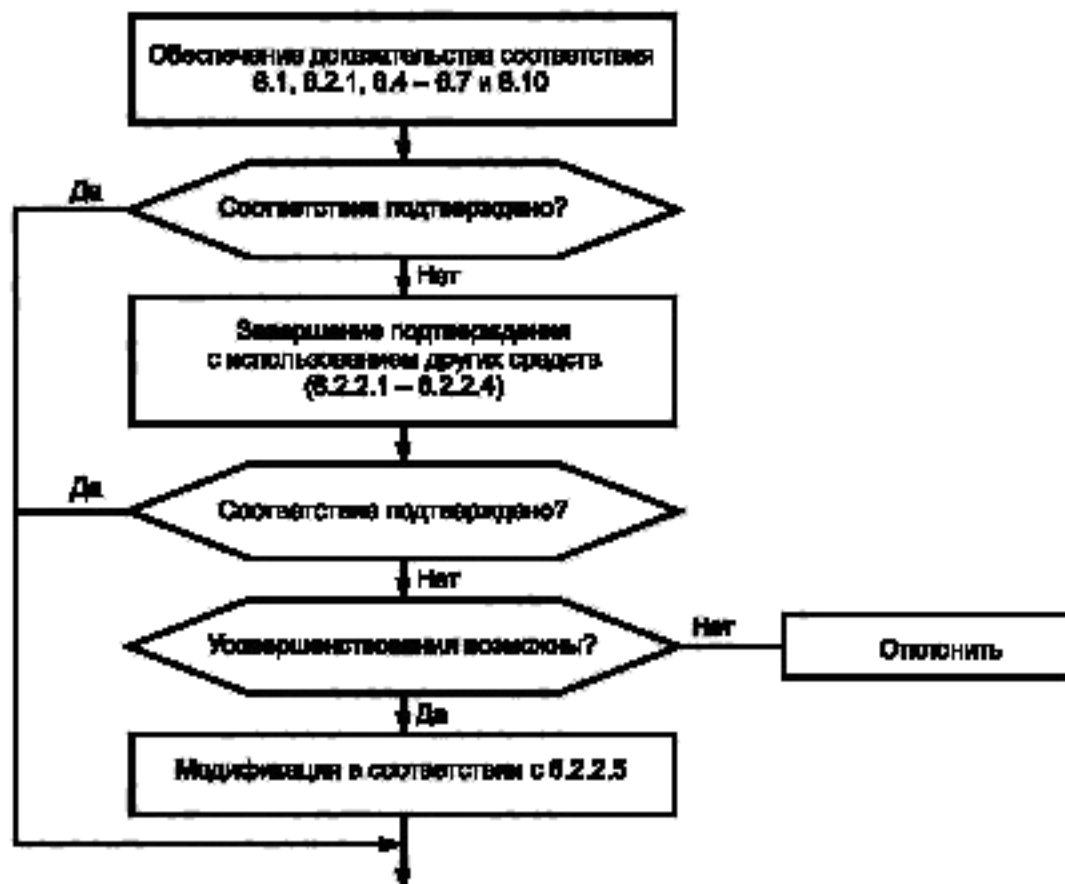
Рисунок 5 — Алгоритм проверки корректности ранее разработанного программного обеспечения для СКУ класса безопасности 2
