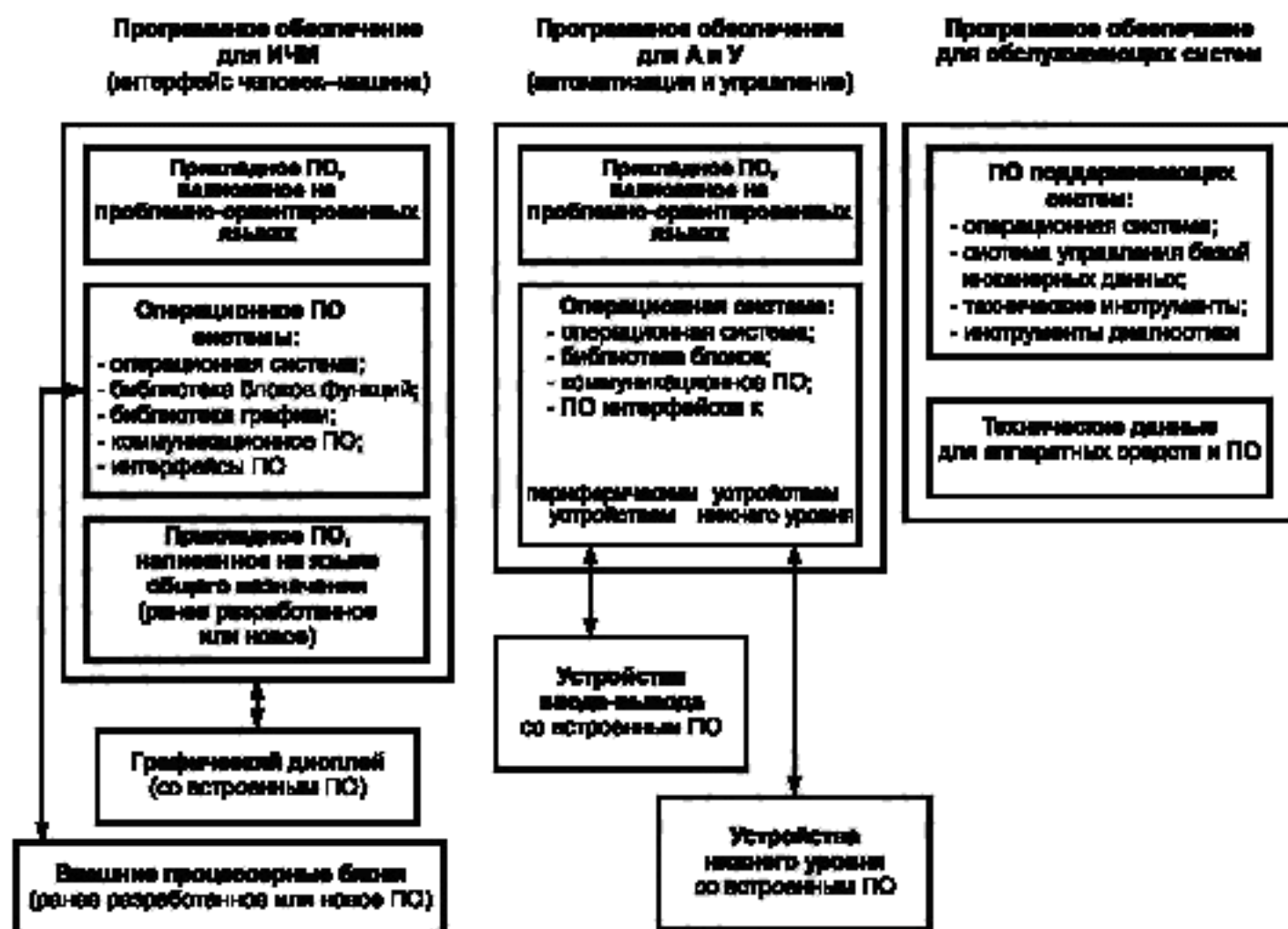
Рисунок 1 — Типичные части программного обеспечения в компьютерных СКУ
